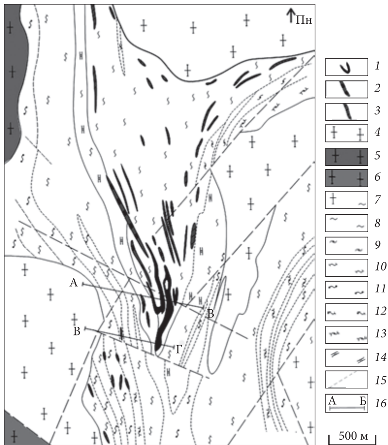
Рис. 1. Геологічна карта Шевченківського родовища. Пегматити: 1 — альбіт-сподуменові; 2 — альбіт-мікроклінові, альбітові; 3 — мікроклінові, мікроклін-олігоклазові керамічні. Граніти: 4 — мусковіт-біотитові; 5 — біотитові; 6 — амфібол-біотитові меланократові, гранодіорити; 7 — мігматити біотитові. Кристалічні сланці: 8 — біотитові; 9 — амфібол-біотитові; 10 — мусковіт-біотитові з кордієритом і силіманітом; 11 — гранат-біотитові з кордієритом і силіманітом; 12 — гранат-мусковіт-біотитові; 13 — біотит-піроксен-амфіболові; 14 — кальцифіри скарновані; 15 — розломи; 16 — лінії геологічних розрізів
